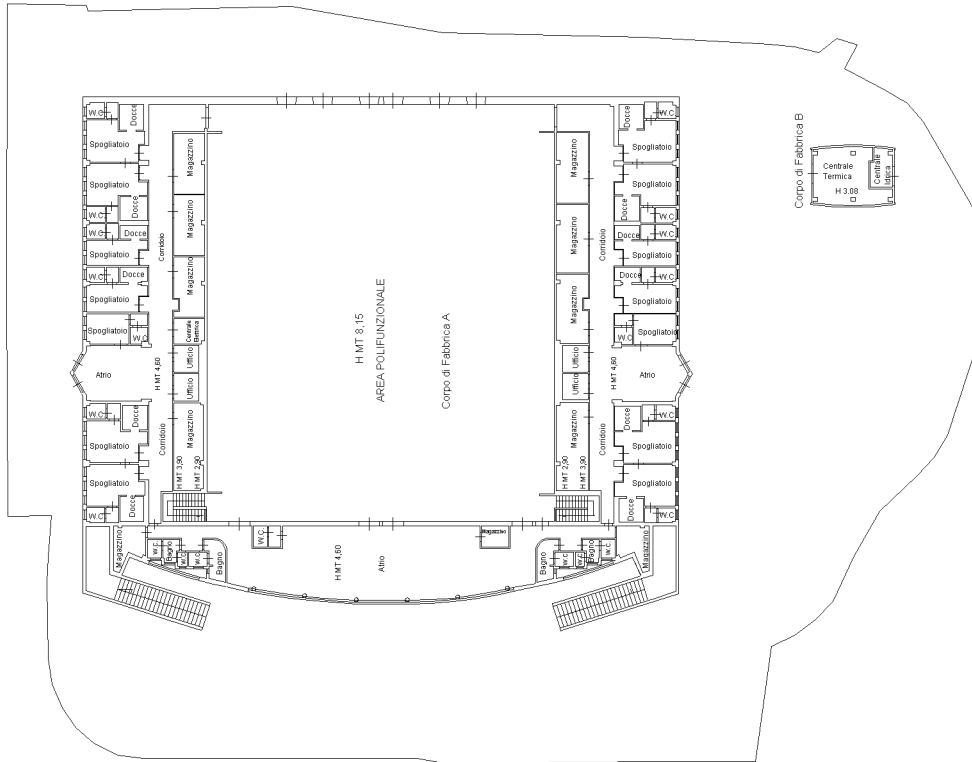
Pianta Piano Terra Palestra Polifunzionale
